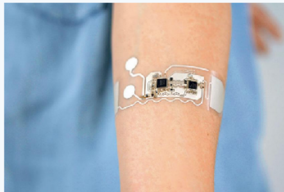
ElasticECG: Rolle zu Rolle (R2R) hergestellter, dehnbarer, energieeffizienter EKG-Sensoren. © VTT
